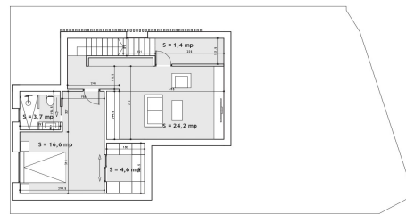
PLANTA SÓTANO
