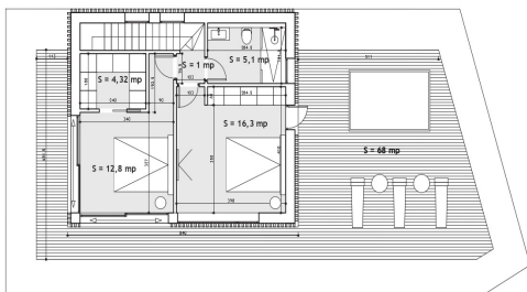
PLANTA ALTA
